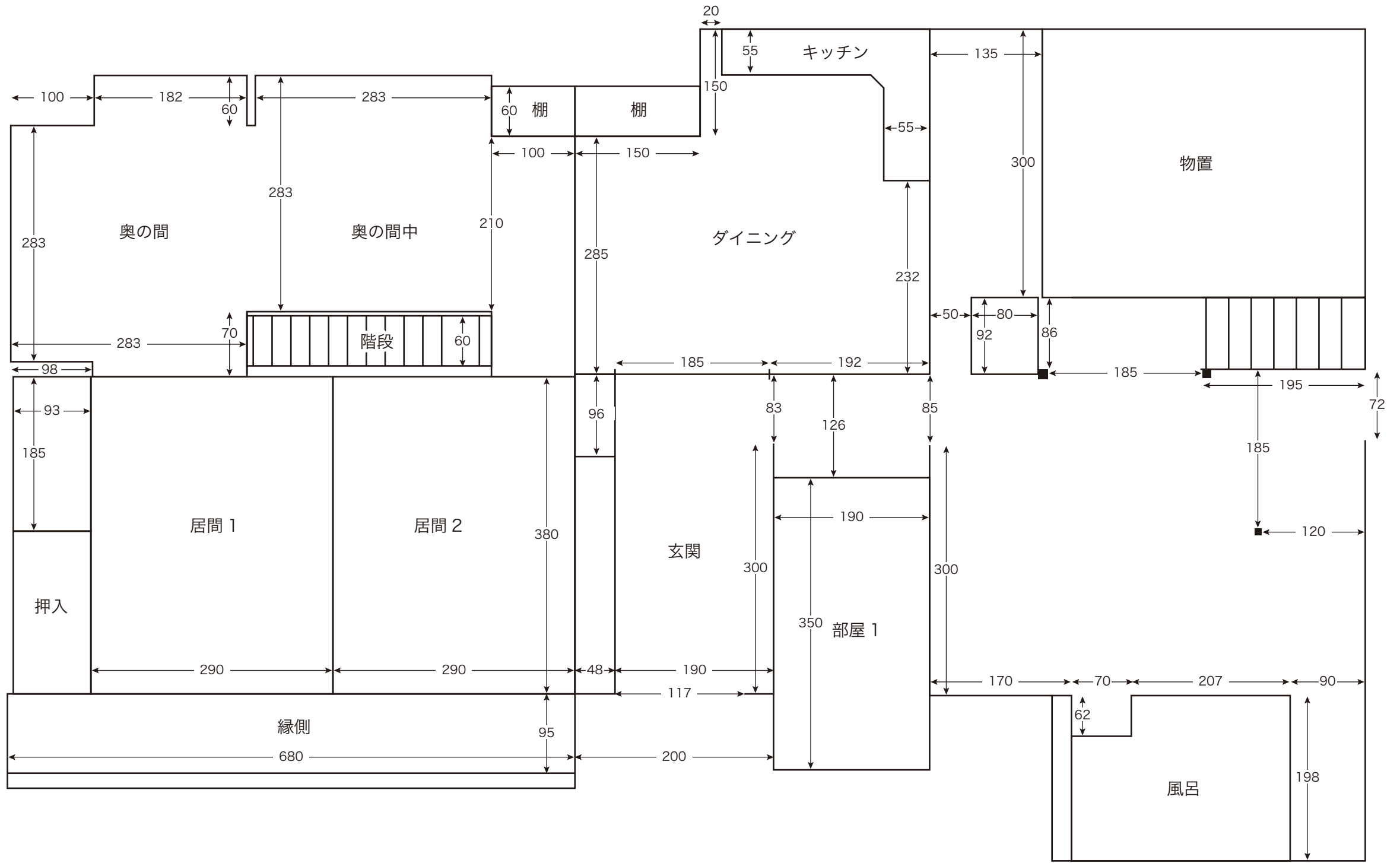
青い家 1階上面図
